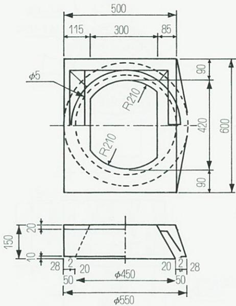
上部側塊
