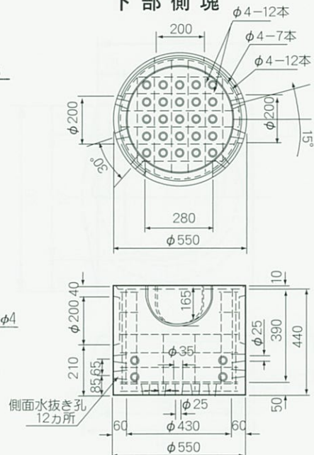
下部側塊
