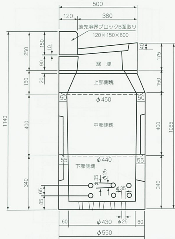
組立図
