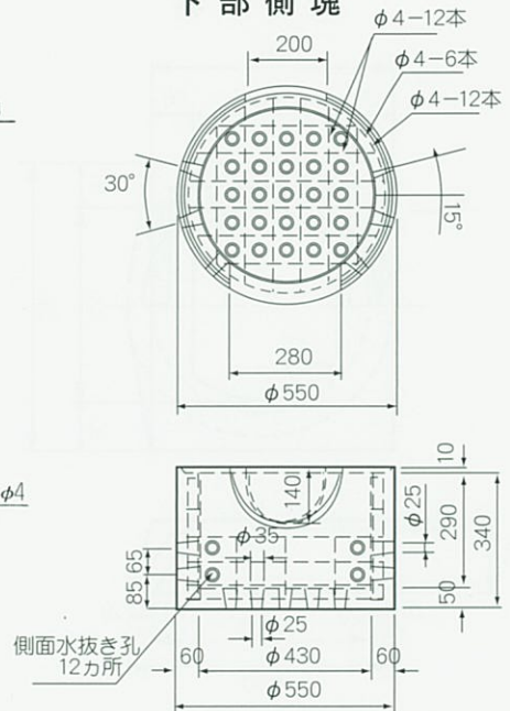
下部側塊
