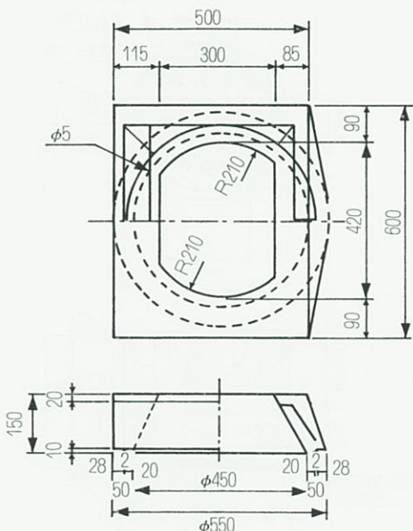
上部側塊
