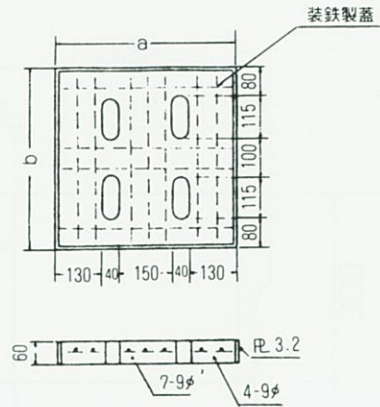
ふ た
