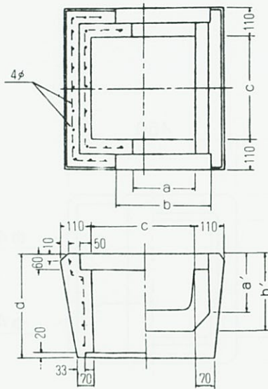
上部側塊
