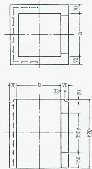
下部側塊
