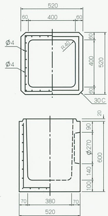
下部側塊
