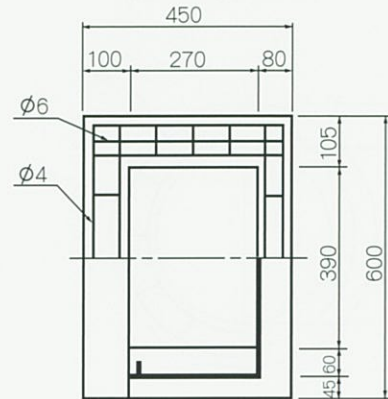
縁塊
