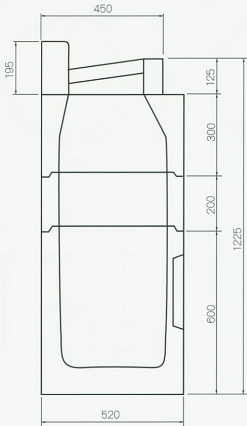
組立図
