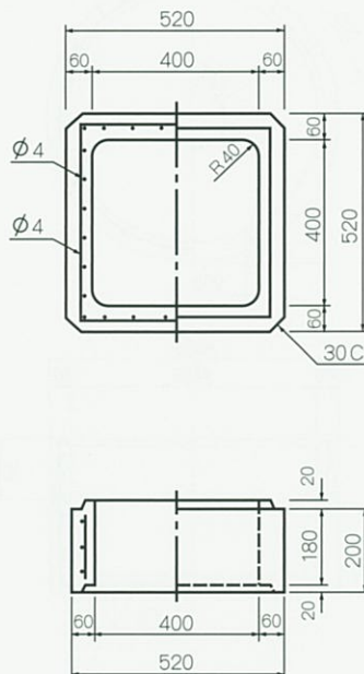
中部側塊
