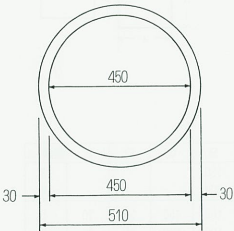
丸半改良ます φ450 × 150
