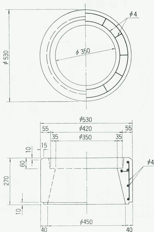
上 部 側 塊
