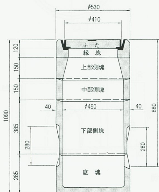
組立図
