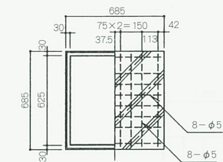
底 版
