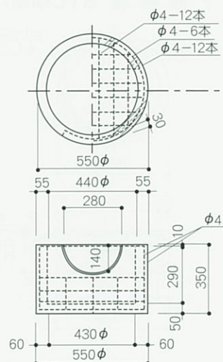
底 塊 (LMM)
