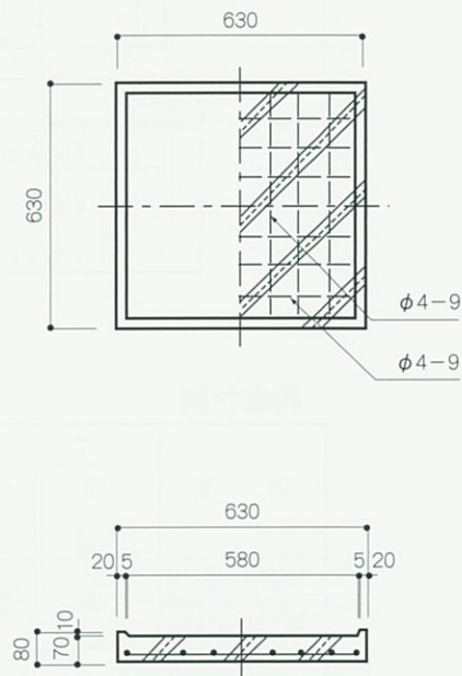
底 版
