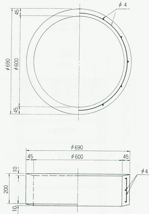
中部側塊
