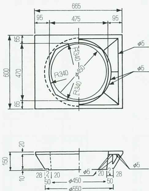
上 部 側 塊
