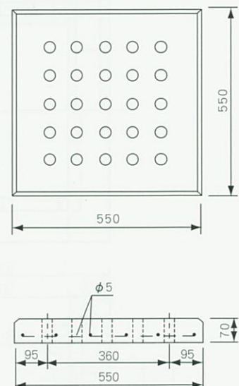
底 塊
