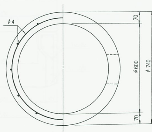
丸 3 - 3 号
