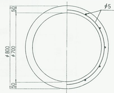
中部側塊 B
