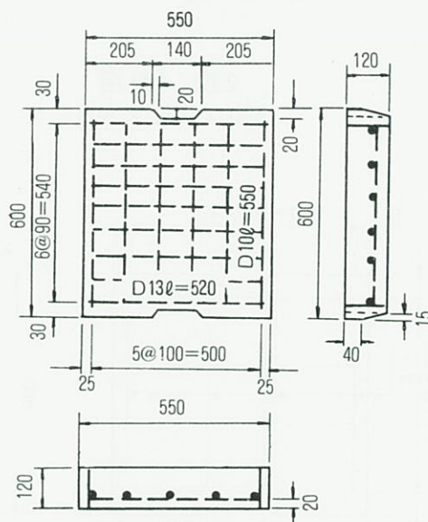
3 種 400 用 (郊外地型)
