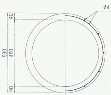
中部側塊
