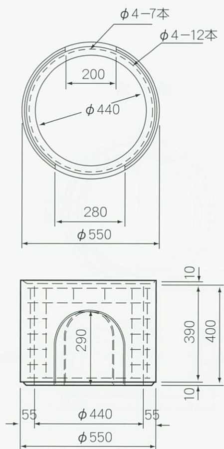
中部側塊
