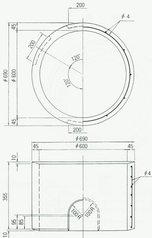
下部側塊
