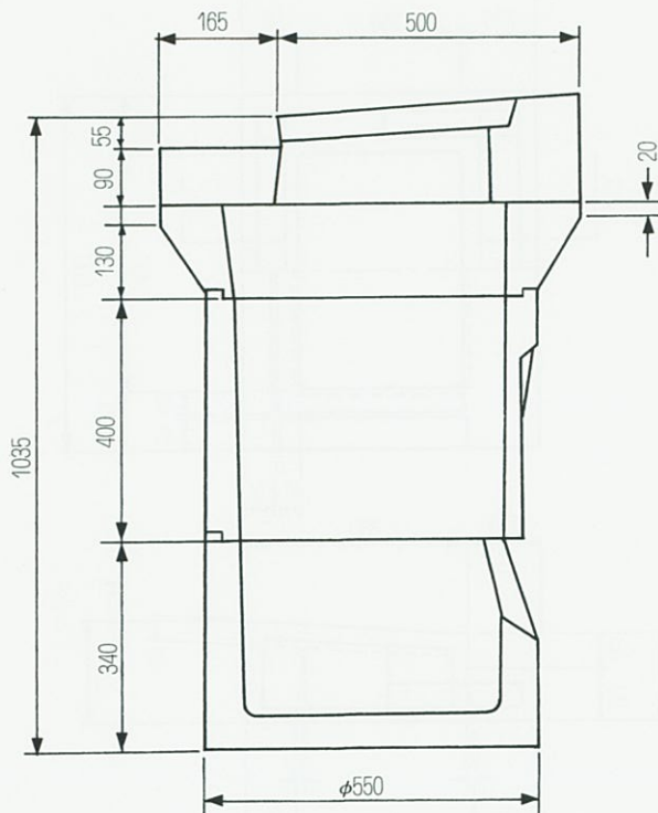
組立図
