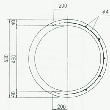
下部側塊
