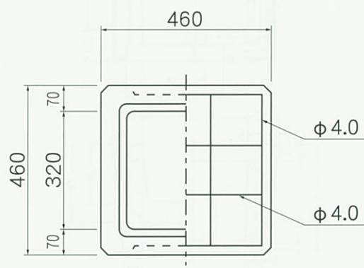
下 部 側 塊
