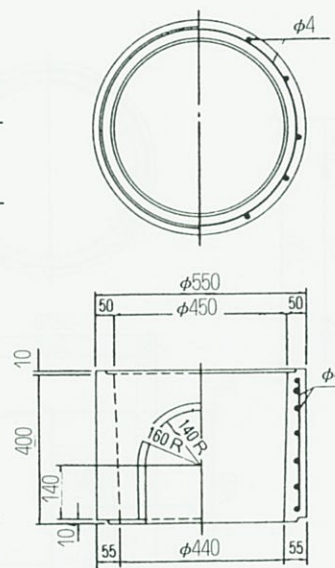
中 部 側 塊
