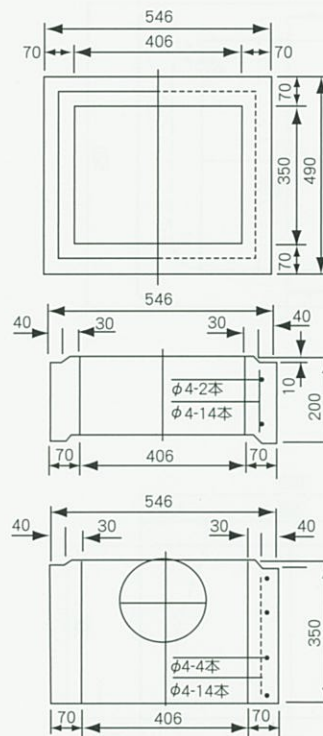
中部側塊
