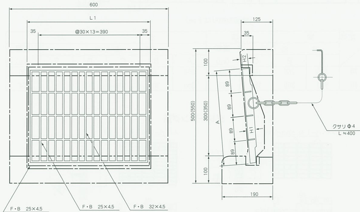
寸法・重量・強度表
