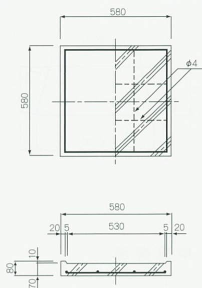
底 版
