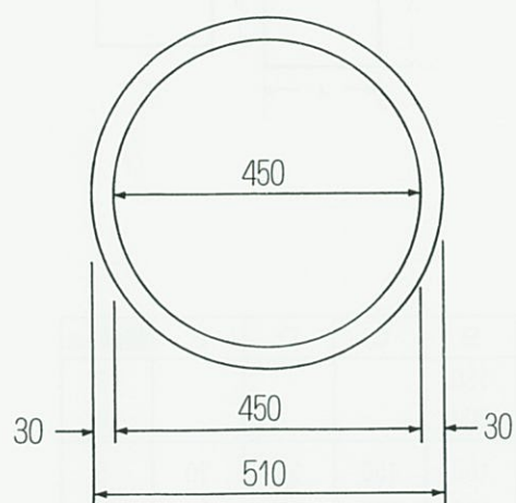
丸半改良ます φ450 × 150
