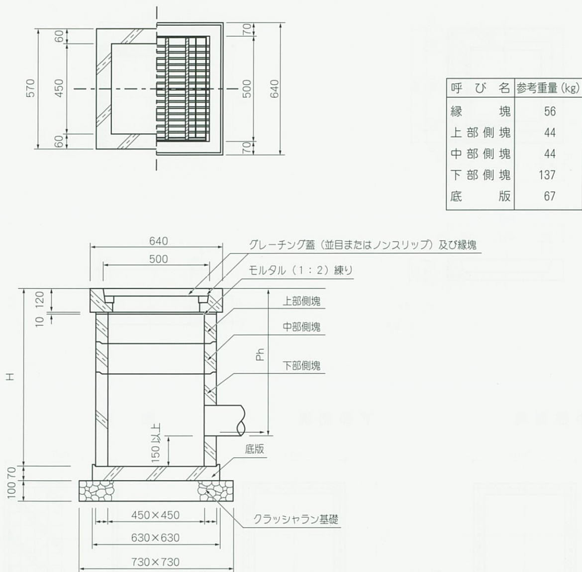
組立図
