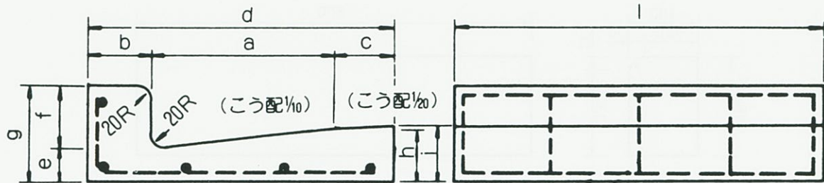
L 形側溝 1 種
