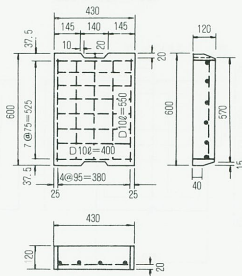
3 種 300 用 (郊外地型)
