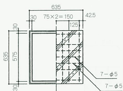
底 版
