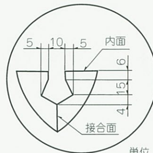
目地部詳細図 1種・3種
