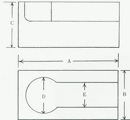
樋受石（モルタル）
