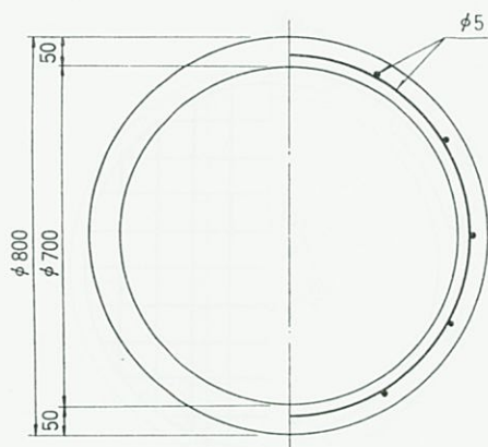
中部側塊 A
