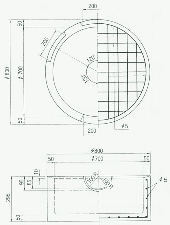
底塊
