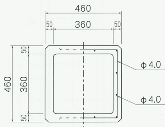
上 部 側 塊
