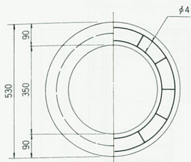
上部側塊
