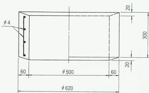
丸 2 - 1 号
