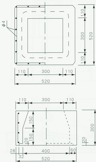
上 部 側 塊
