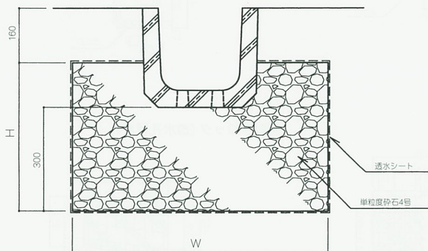
据付寸法表
