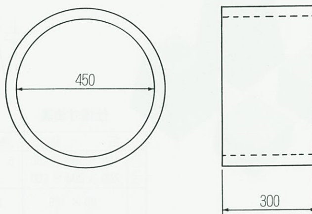
丸改良ます φ450 × 300
