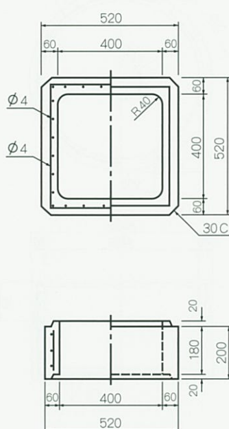
中 部 側 塊
