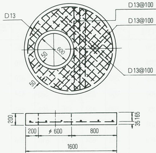
第2種B型
