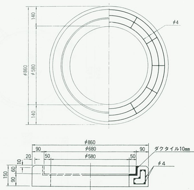
縁 塊
