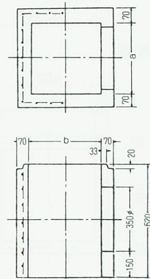
下 部 側 塊
