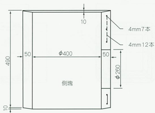
下部側塊
