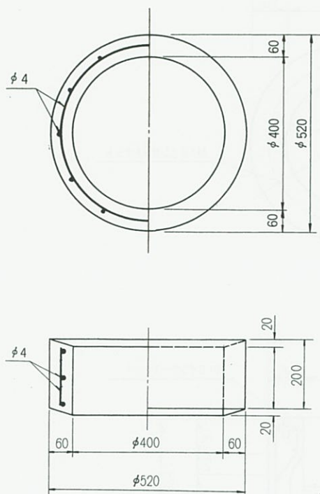
丸 1 - 1 号
