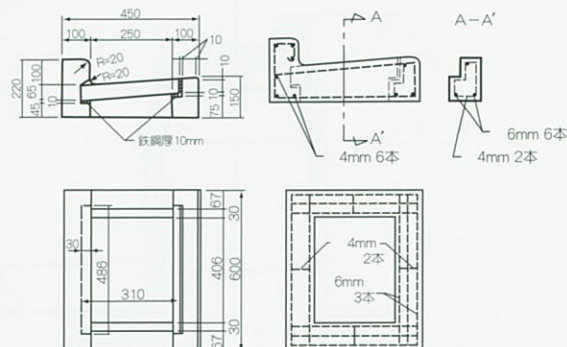
縁塊
