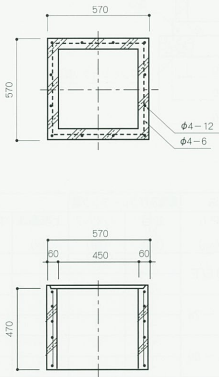
下 部 側 塊
