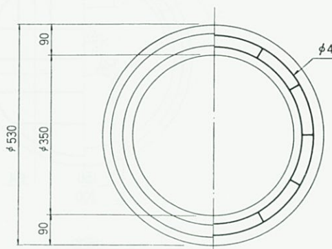
上部側塊
