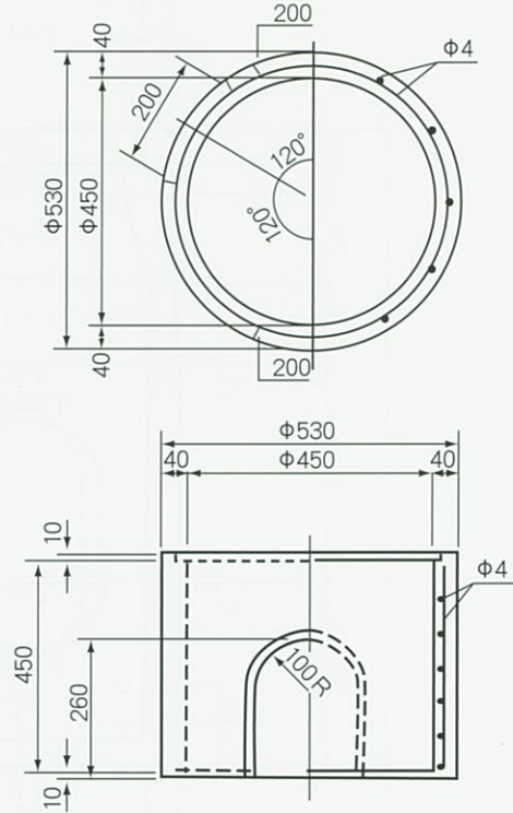
下部側塊
