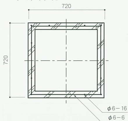
下 部 側 塊
