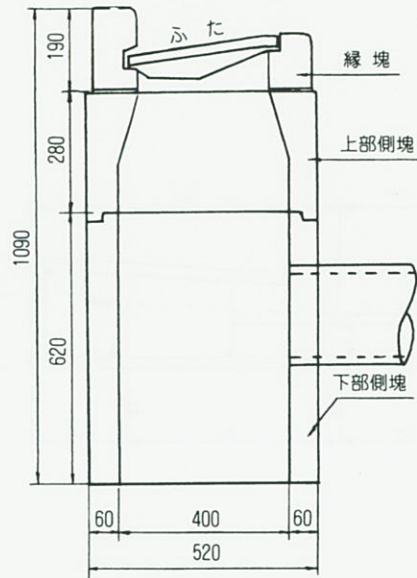
組立図
