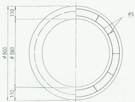
上部側塊
