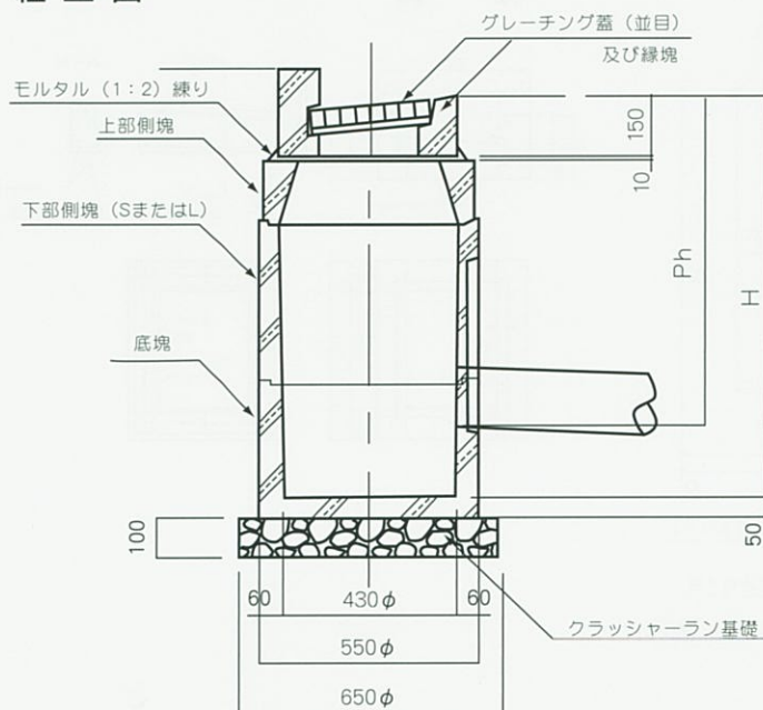
組立図
