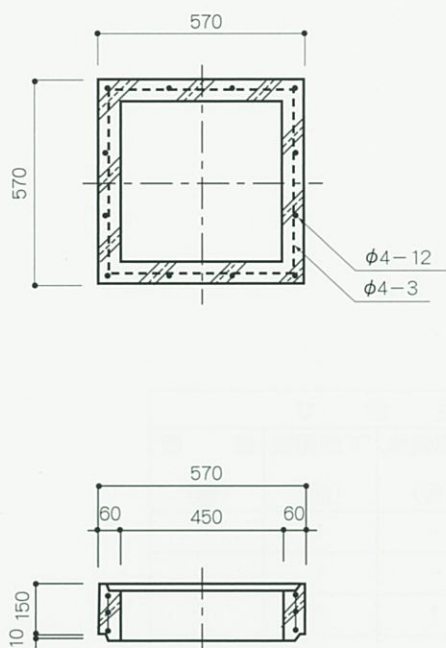
中 部 側 塊
