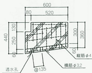
側面図
