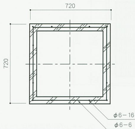
上 部 側 塊
