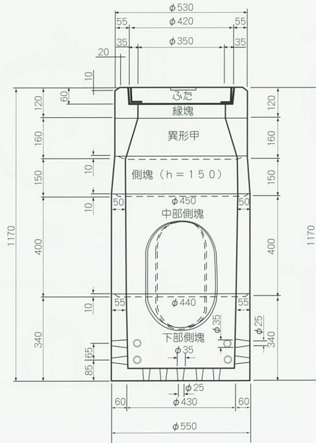
ふ た
