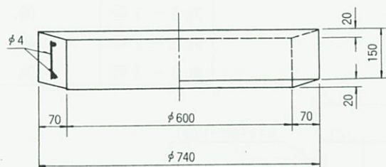
丸 3 - 2 号
