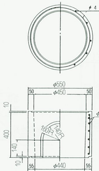
中部側塊
