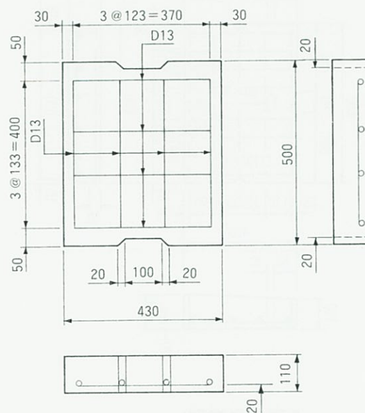
2 種 300 用 430 × 110 × 500
