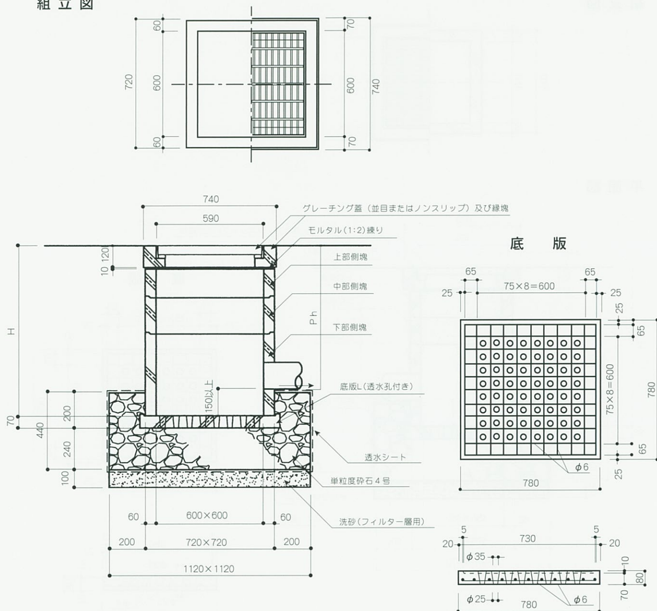
組合せ表
