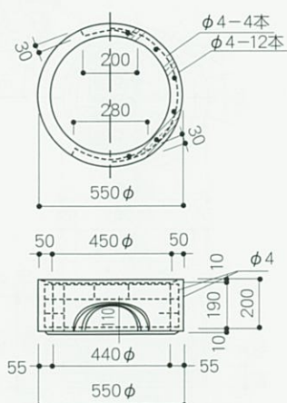
下 部 側 塊 S (LMM)
