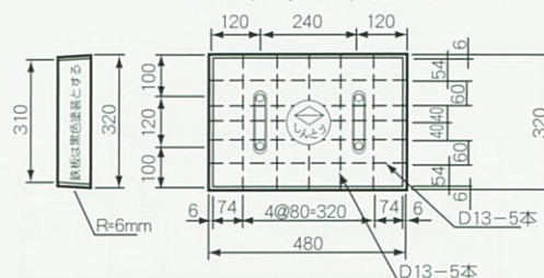
コンクリートふた
