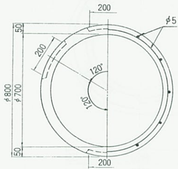
下部側塊
