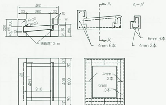
縁 塊
