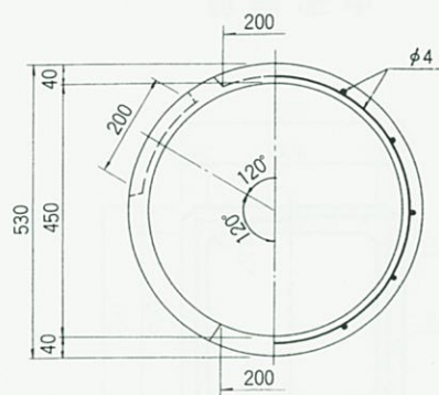
底塊
