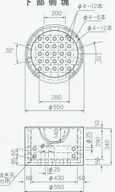
下部側塊
