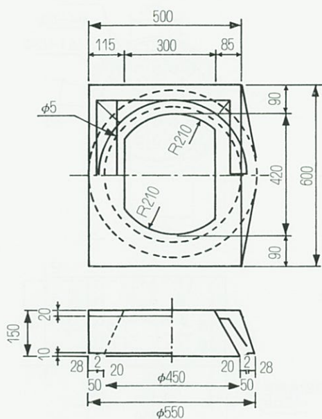
上部側塊
