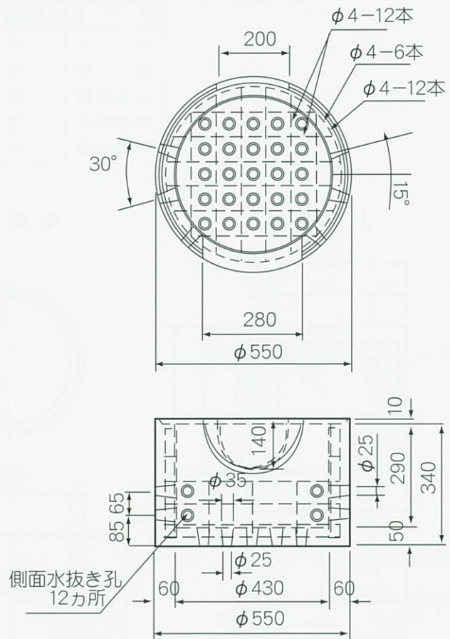
下部側塊
