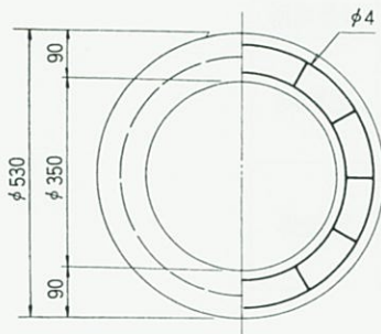
上部側塊
