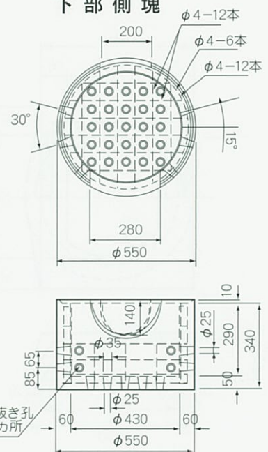
下部側塊
