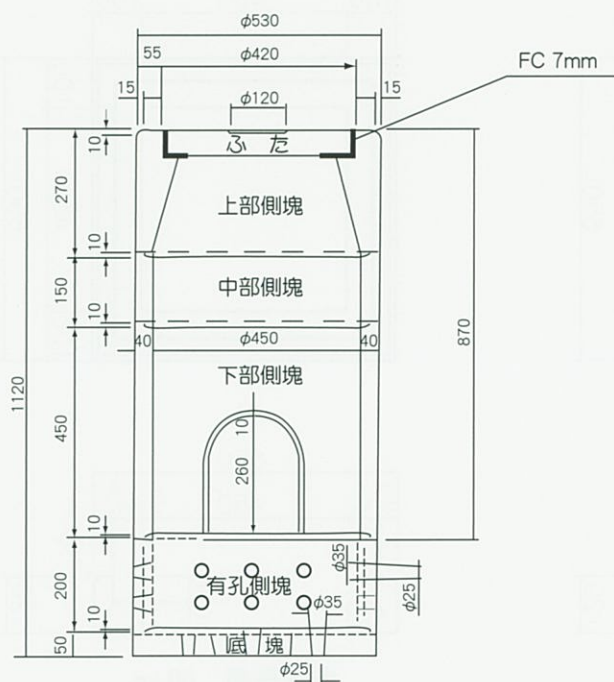
組立図
