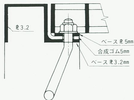
ボルト取付方法
