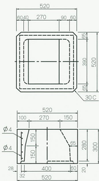
上 部 側 塊
