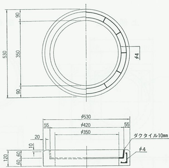
縁 塊
