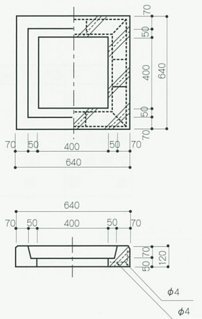
縁 塊
