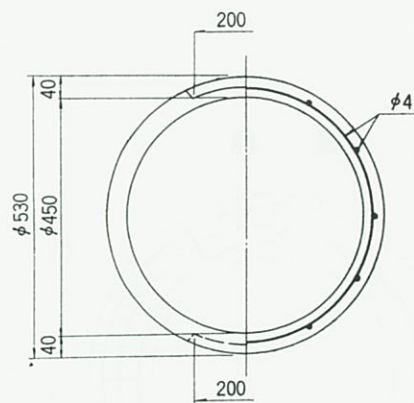
下部側塊
