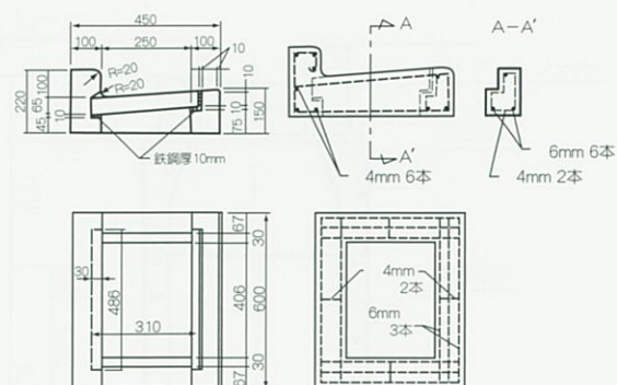
縁 塊
