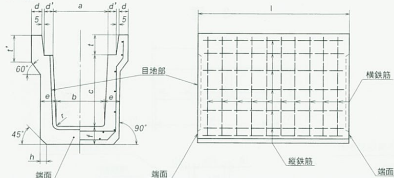
本体の寸法、配筋及び寸法の許容差
