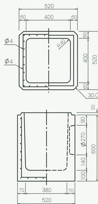
下 部 側 塊
