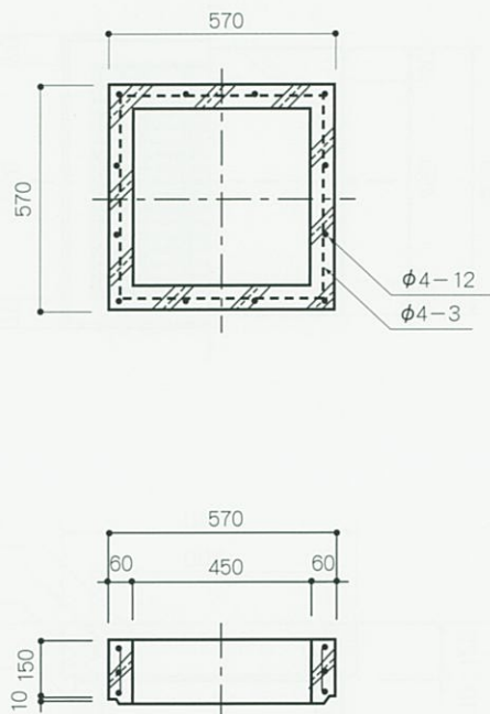
上 部 側 塊
