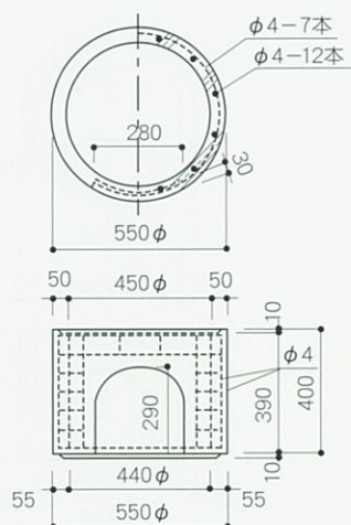
下 部 側 塊 L (LMM)
