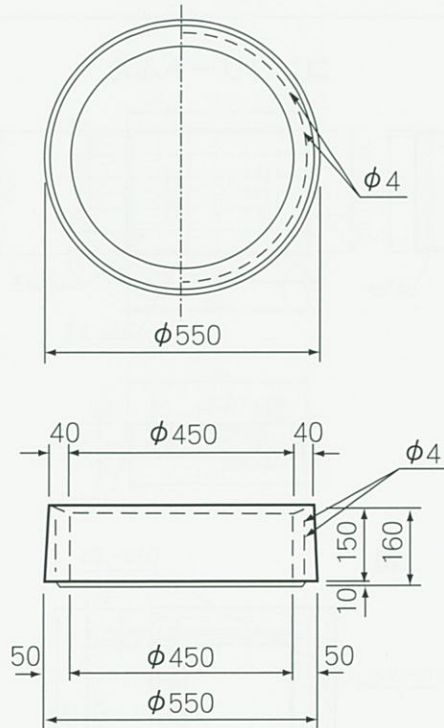
側 塊 (h = 150)
