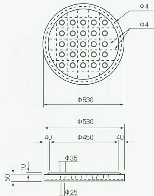
有孔底塊
