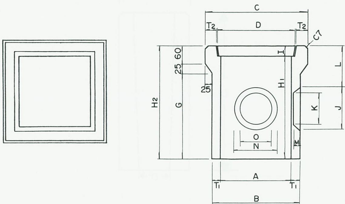
寸法表
