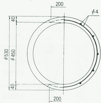
下部側塊
