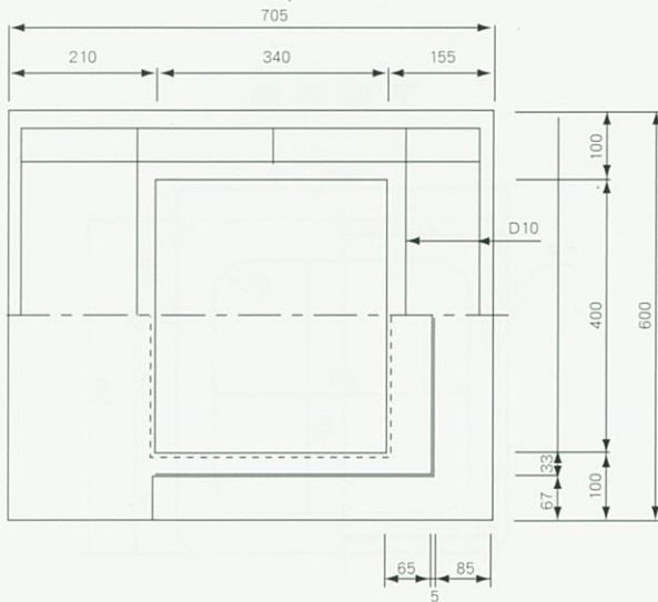
川崎市型街渠ます 155 縁塊頭無し
