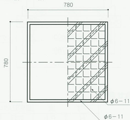
底 版
