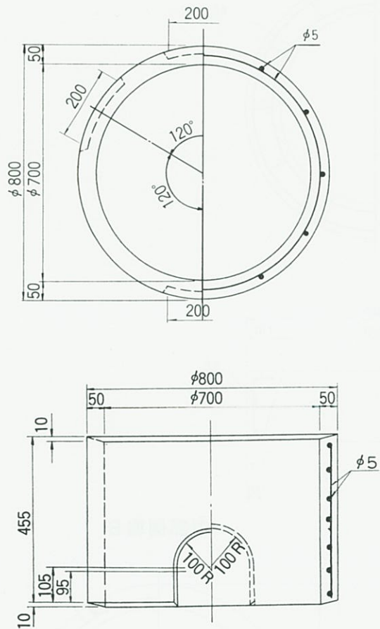
下部側塊
