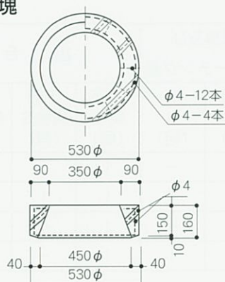
下 部 側 塊 S (LMM)
