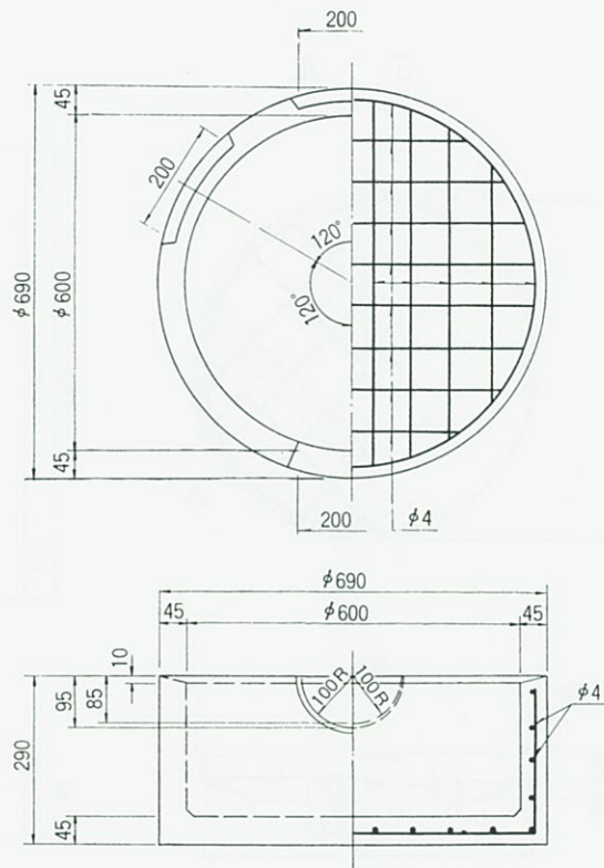
底塊
