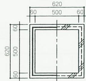
下 部 側 塊
