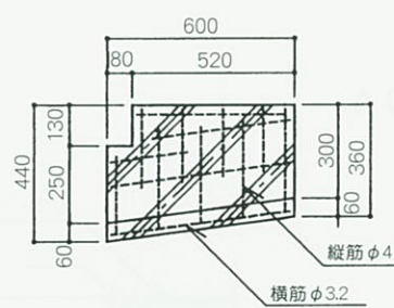
側溝ブロック
