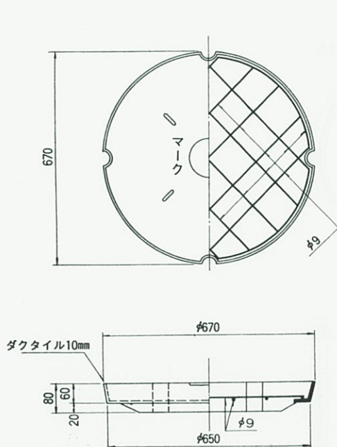
ふ た
