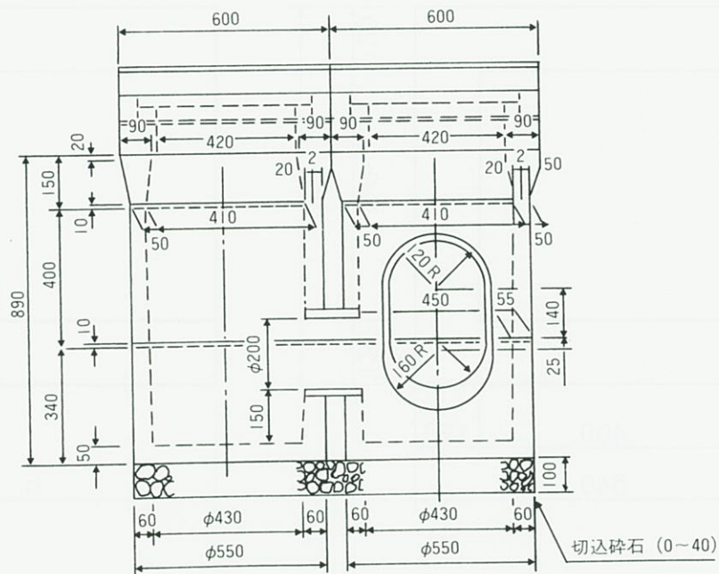
側面図
