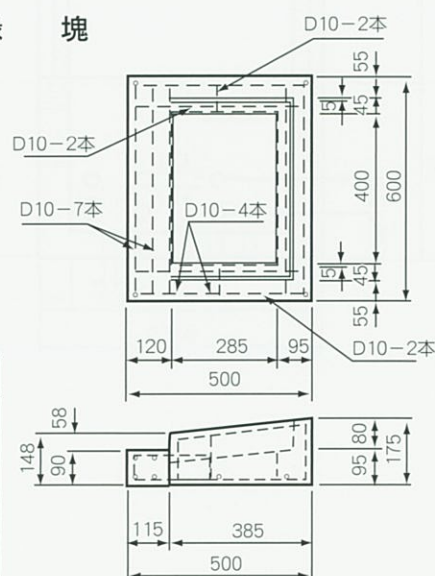
下部側塊
