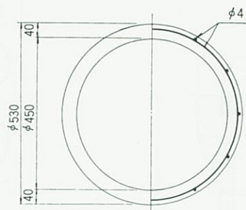
中部側塊
