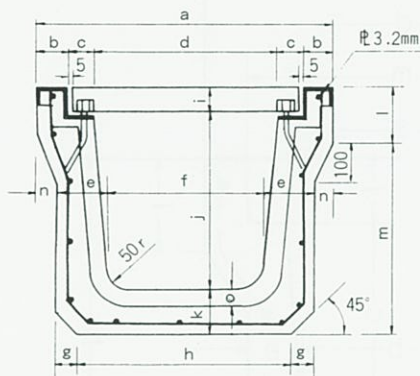
横断用U形
