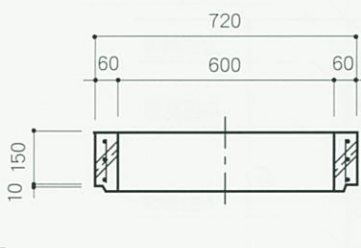
底 版
