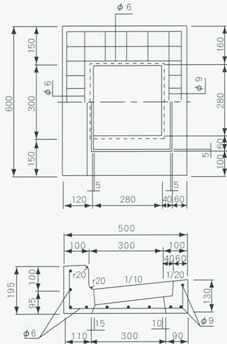
B 型 縁 塊
