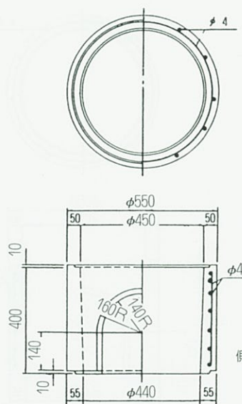
中部側塊
