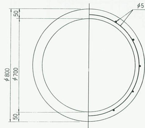
中部側塊 B
