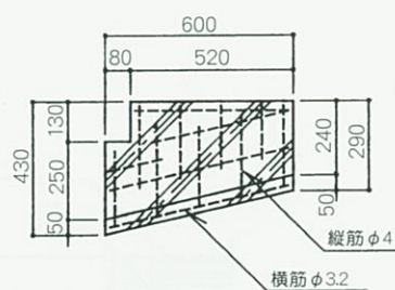
側溝ブロック
