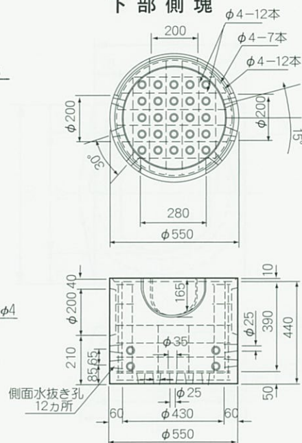
下部側塊
