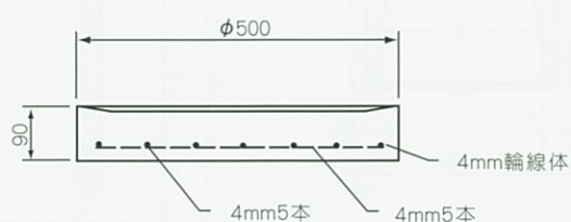
底 版
