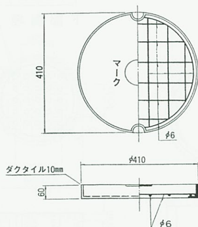
ふ た
